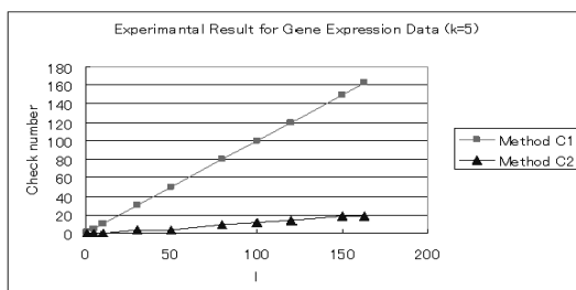
図 21 人工データの実験結果 ( k=5 )
