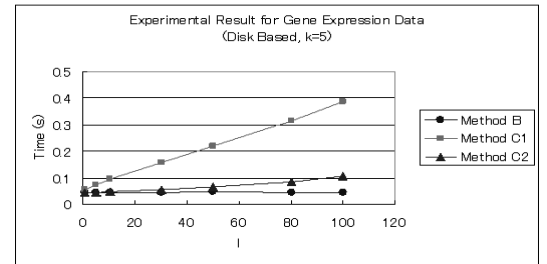
図 22 ディスクベースの遺伝子発現量データの実験結果 ( k=5 )
