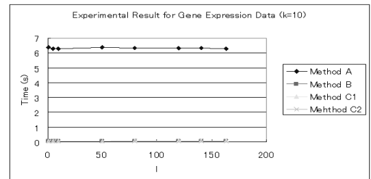
図 15 人工データの実験結果 ( k=10 )
