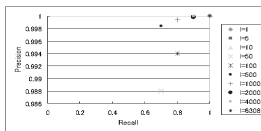
図 9 人工データの実験結果 ( k=10 )
