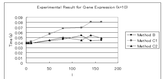
図 16 人工データの実験結果 ( k=10 )
