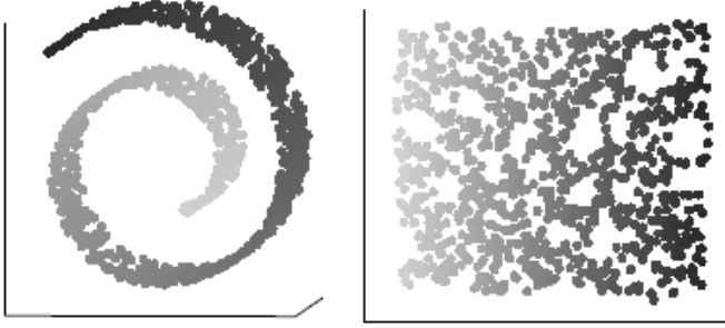
図 2 Tenenbaum のロールケーキデータとその 2 次元に圧縮した結果 ([7] から)
