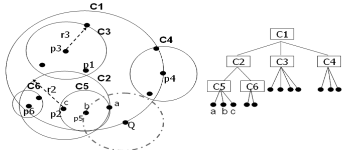
図 3 M-Tree の例
