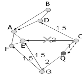
図 7 削除処理の例
