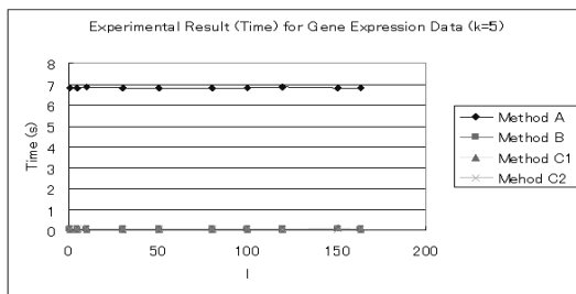
図 19 人工データの実験結果 ( k=5 )
