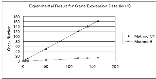
図 17 人工データの実験結果 ( k=10 )
