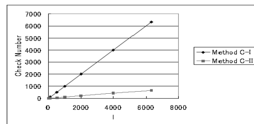
図 12 人工データの実験結果 ( k=10 )
