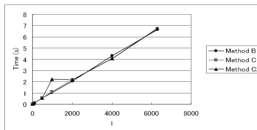
図 11 人工データの実験結果 ( k=10 )
