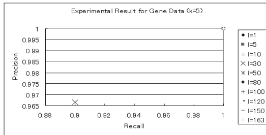
図 18 人工データの実験結果 ( k=5 )
