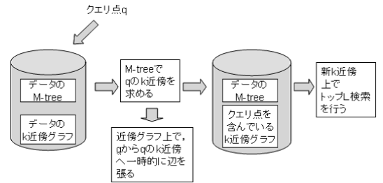
図 4 クエリの処理の流れ
