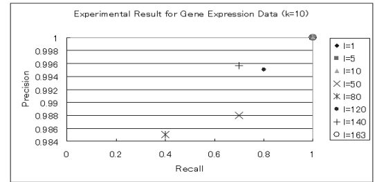
図 14 人工データの実験結果 ( k=10 )
