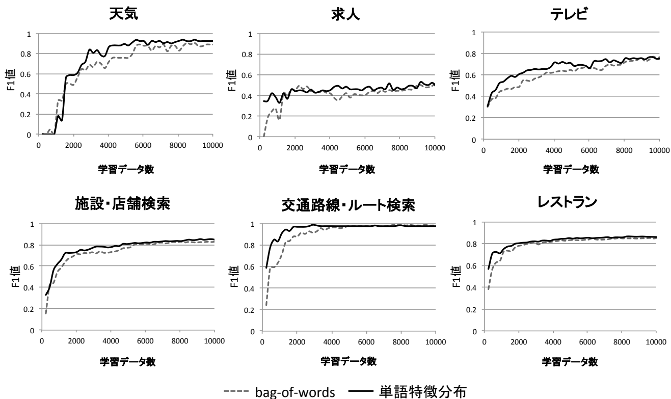
図 5 カテゴリ別の分類精度と学習データの質問文数の関係。
