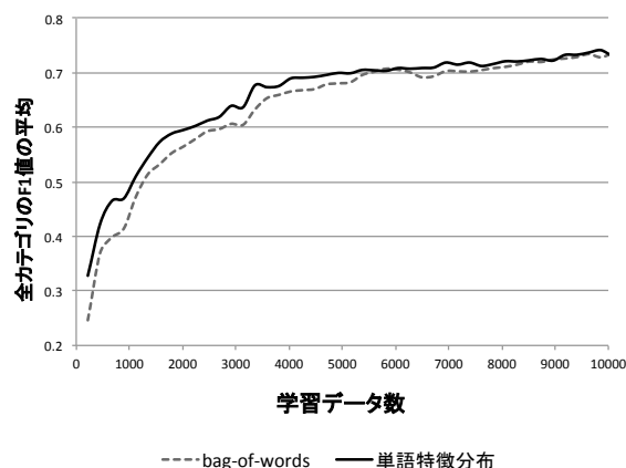
図 4 学習に用いる質問文数と分類精度の関係。
