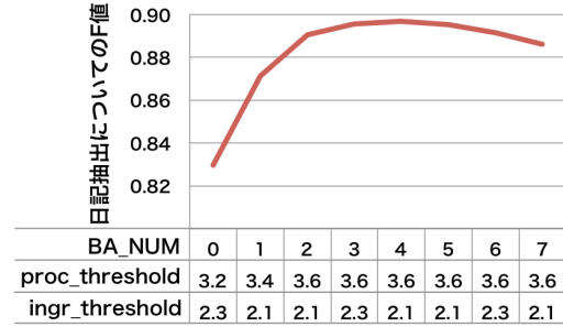
図 5 日記抽出結果の F 値の変化
