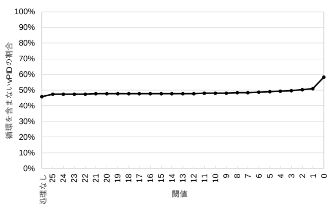
図10 ノード集約方式2に於ける閾値の変化に伴う循環を含まないvPID割合の推移
