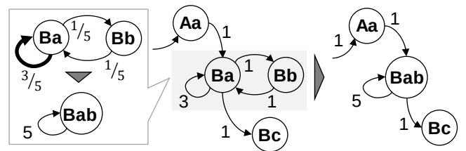
図 5 ID の遷移頻度を活用したノード集約方式の模式図
