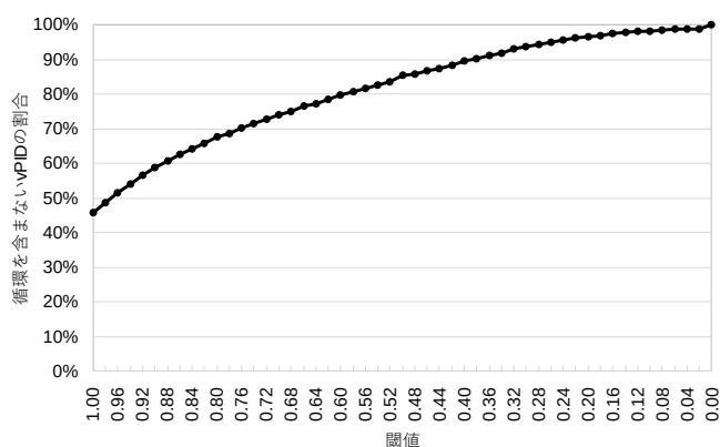
図9 ノード集約方式1に於ける閾値の変化に伴う循環を含まないvPID割合の推移
