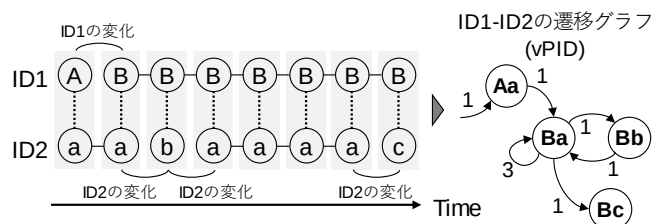
図 3 ID1-ID2 の遷移グラフ (vPID) の作成方法
