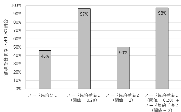
図 11 ノード集約方式ごとの循環を含まない vPID 割合の比較グラフ
