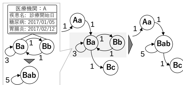
図 7 疾患情報を活用したノード集約方式の模式図
