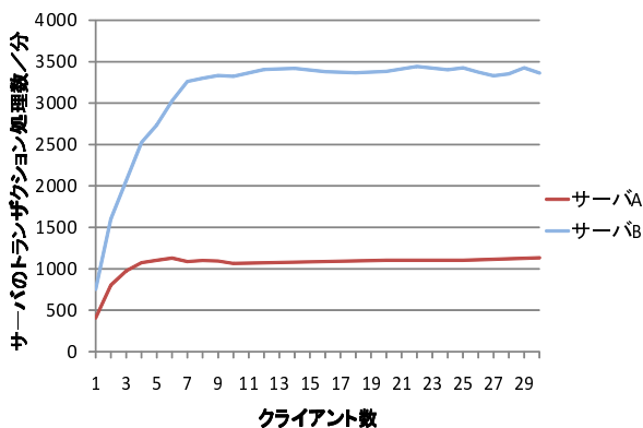
図 4 サーバの負荷実験
