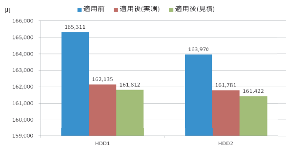
図 7 省電力状態適用による TPC-H 実行時消費エネルギー比較
