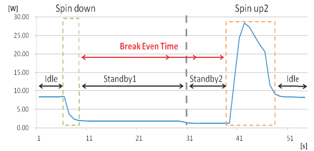
図 4 ディスクの状態遷移における消費電力と Break-Even Time(HDD1)
