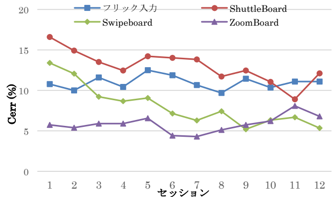
図 4.2 各手法の各セッションにおける平均 Cerr
