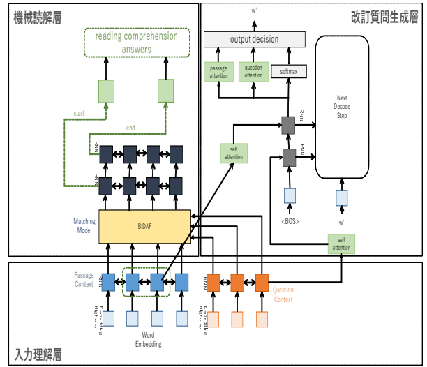
図 3 機械読解と改訂質問生成のマルチタスクモデル
